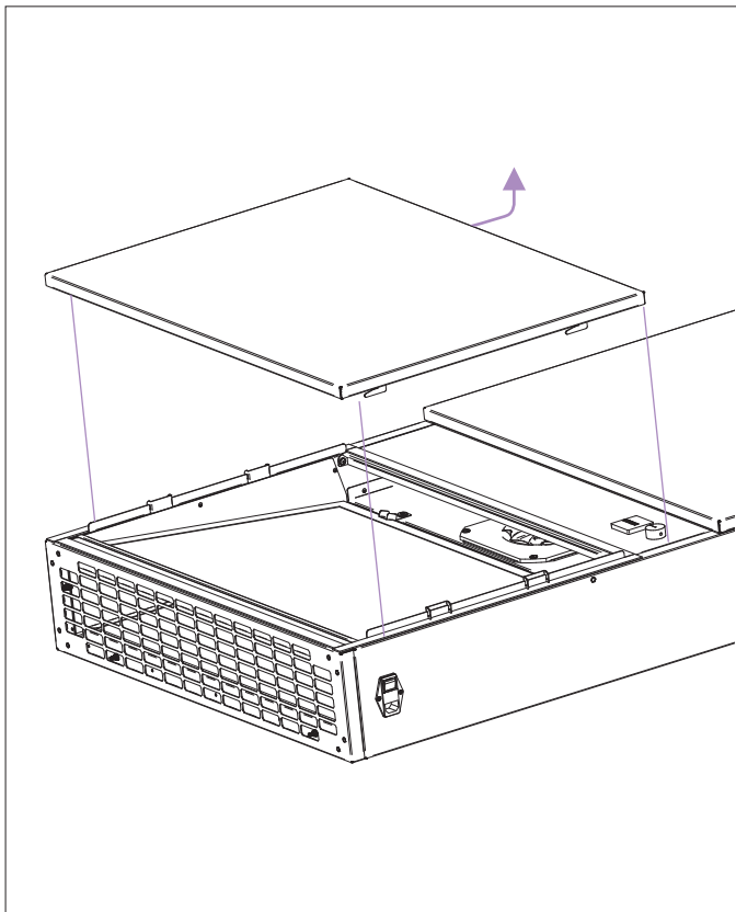
Abnehmen der Filtertür nach Entfernung der Sicherungsschraube.
